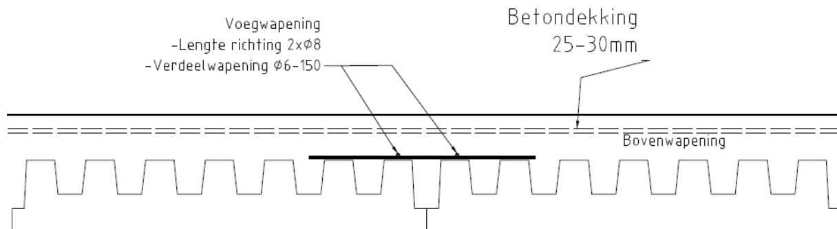
Afbeelding 2: Doorsnede opstort aslast kelderdekken met wapening.
